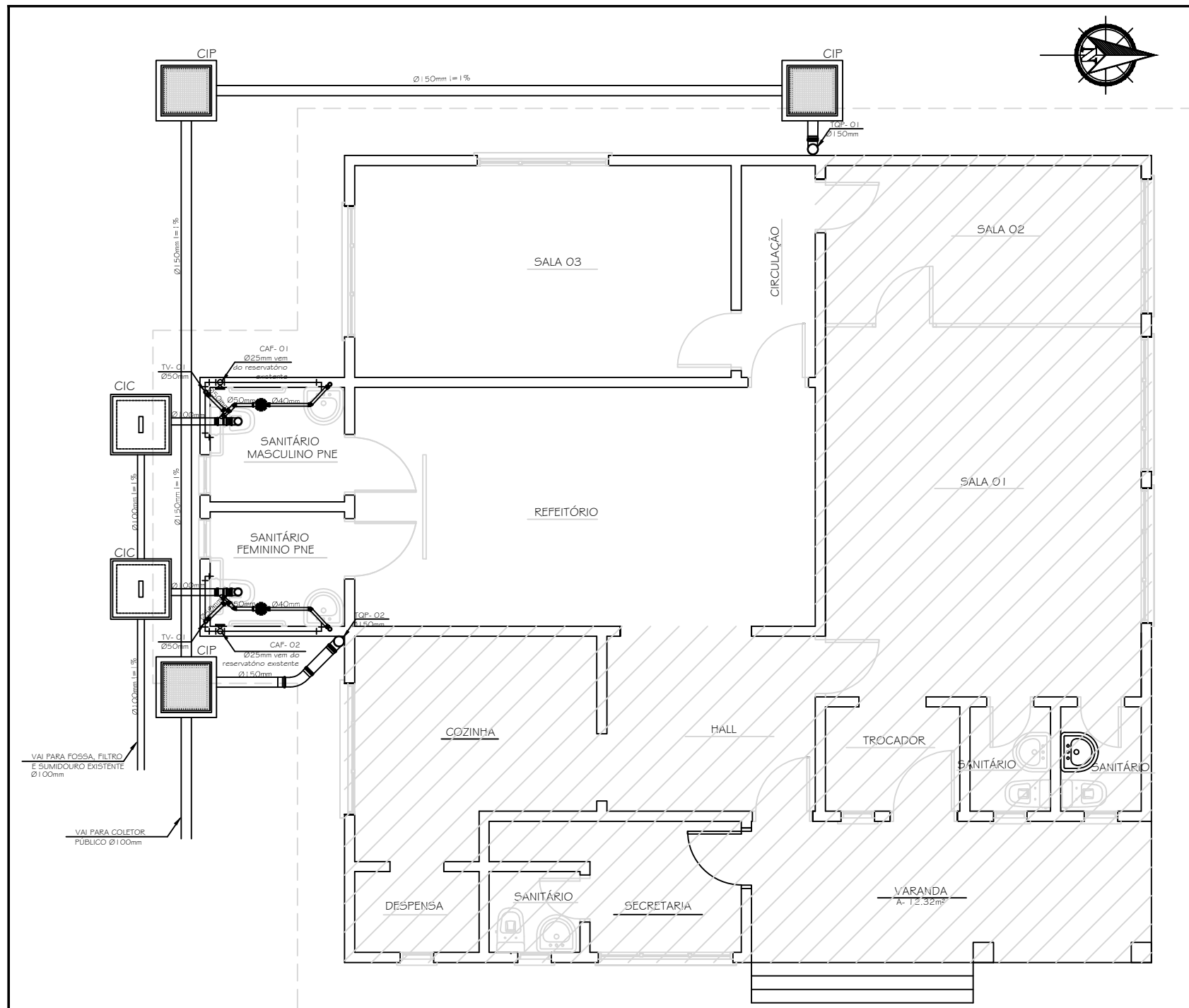
PLANTA PROJETO HIDROSSANITÁRIO ESC.: 1/75
