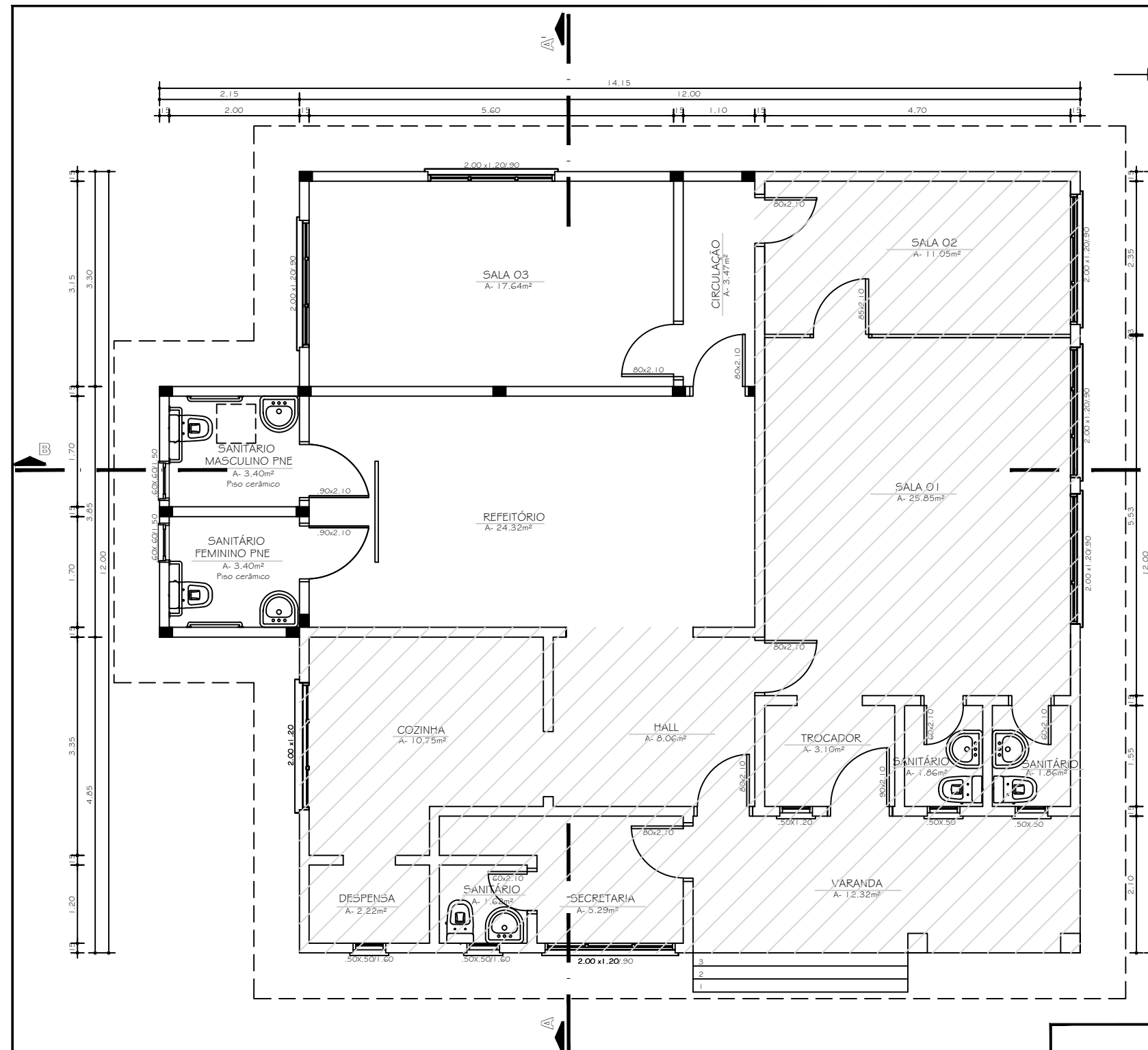
PLANTA BAIXA ESC.: 1/75
